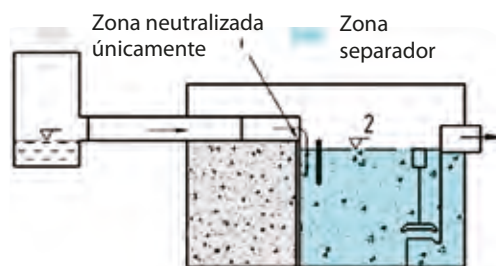
Esquema de principio de un separador (con cámara de separación única):
