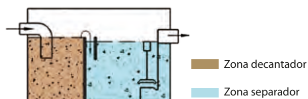
Esquema de principio de un separador de hidrocarburos combinado con un decantador:
