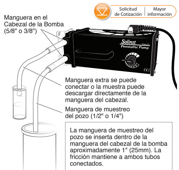
Modelo 410 Configuración de la Bomba Peristáltica
