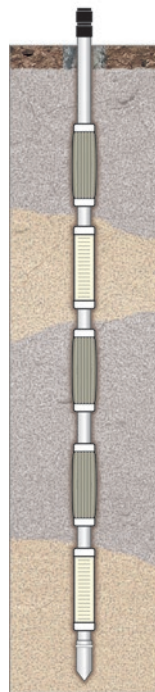
Instalación típica Sistema CMT 3 canales en suelo sedimentario con cartuchos de arena y bentonita
