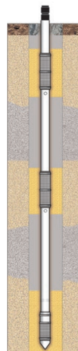
Instalación típica Sistema CMT de 3 ó 7 canales rellena desde la superficie con arena y bentonita
